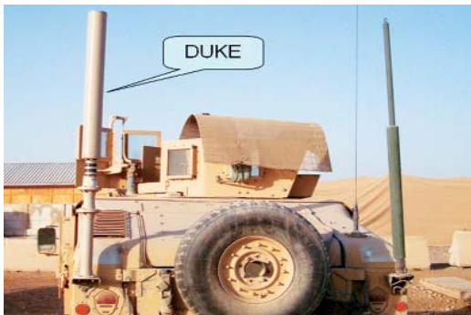
그림 20-16. DUKE 및 RHINO C-IED 시스템
