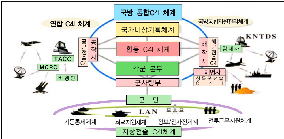
[도표 4-9] 국방통합C4I체계도
